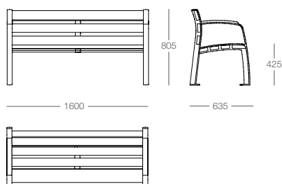
Elegance Confort bench with backrest banc avec dossier Elegance Confort banco com costas Elegance Confort
